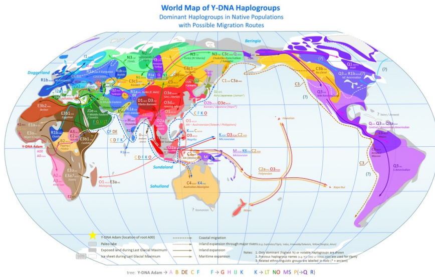
Мапа світової генографії. Автор: Chakazul
